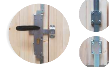
Tablier de lame bois 89 x 27 mm
